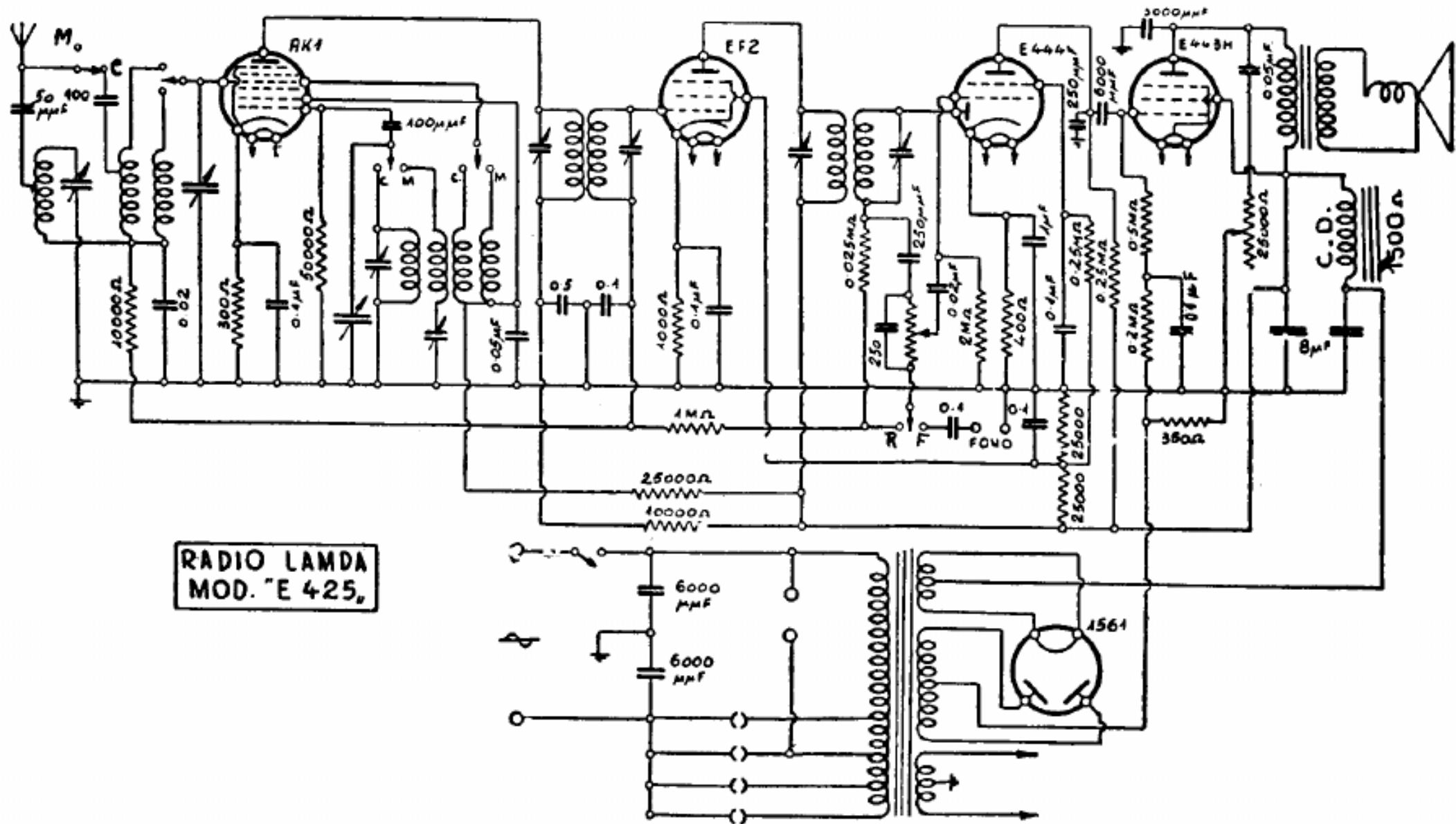
OLIVIERI E GLISENTI. — Modello « Lamda E 425 ». - Produzione 1934. - Media frequenza: 175 kc.
